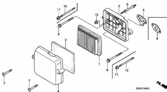
Fig. 6. Se montează reperatele 3, 5, 9, 10, în ordinea corespunzătoare.
